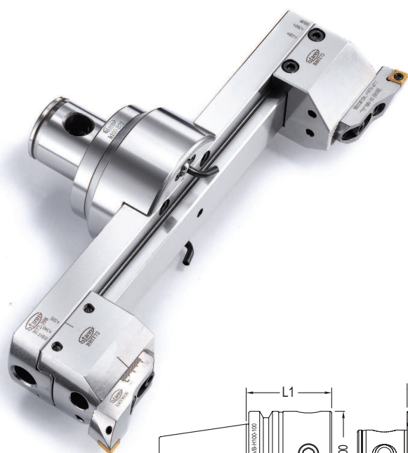
H100 系列-搪孔刀柄 Taper Shank
