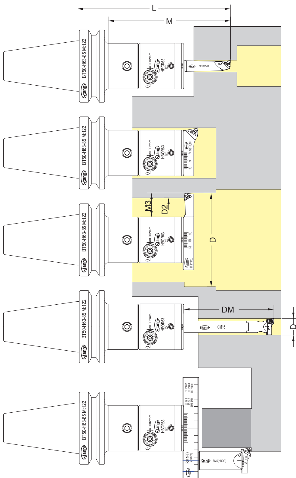
精搪孔刀桿
