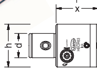
精搪孔刀本體 Body
