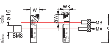
精搪孔刀座 Cutting Insert Holder
